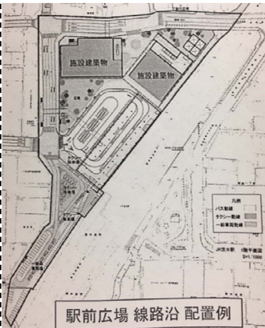
(配置図1)
